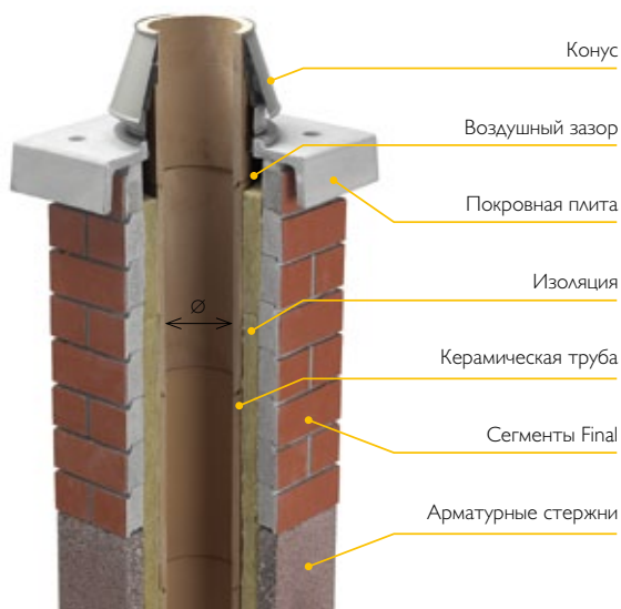
Комплект UNI Final для верхней части дымовой трубы
